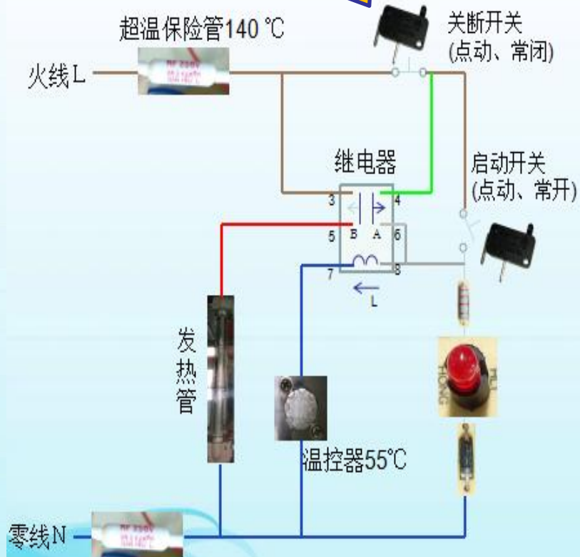
启动开关 (点动型、常开)
