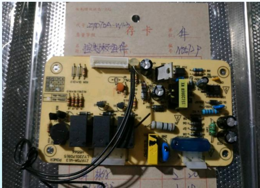
控制板 N05729
