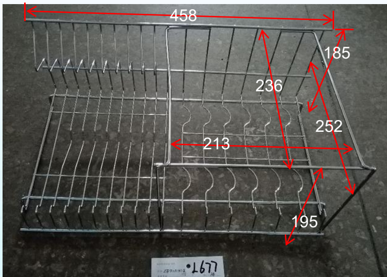
大层架L677
