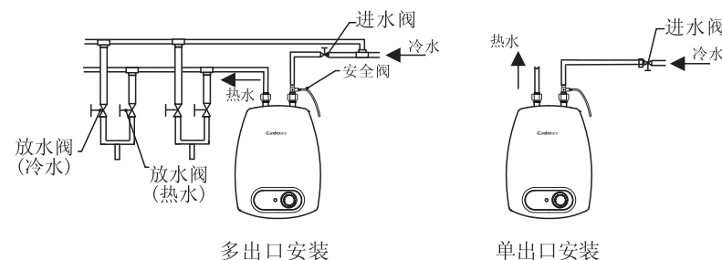
上出水机型
