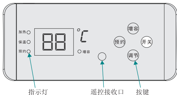
控制盒操作示意图
