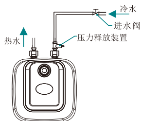
单出口安装
