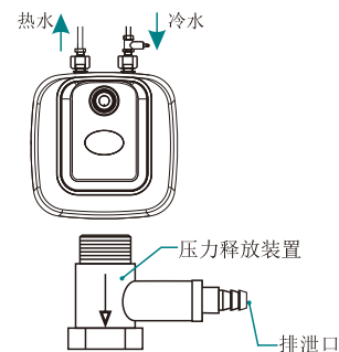
上出水机型安装图
