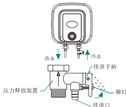
（下出水型压力释放装置放大图）
