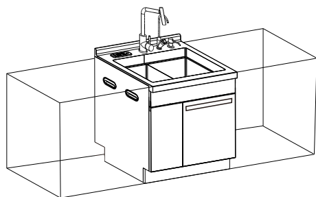
整机与橱柜关系安装示意图
