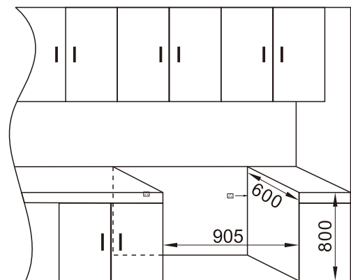
整机与橱柜关系安装示意图
