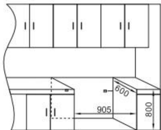
整机与橱柜关系安装示意图
