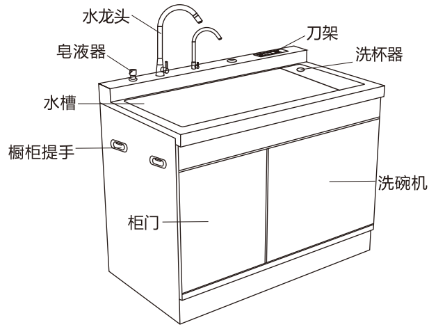
JCS-1050-XD9安装示意图
