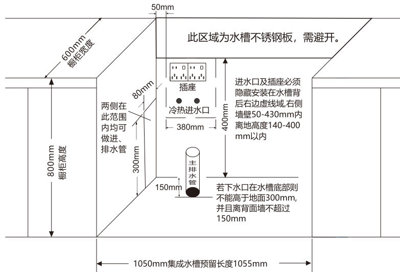
集成水槽（电源、给水、排水）安装示意图
