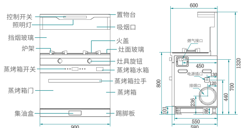
(此图为示意图，具体以实物为准！单位：mm)
