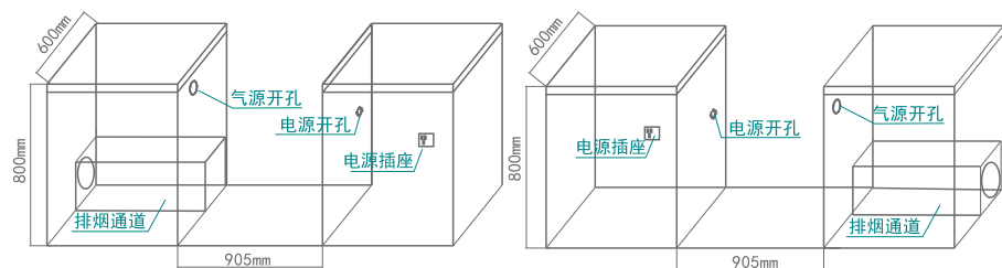
(图一 排烟管左边安装图)
