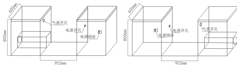
(图二 排烟管左右安装图)
