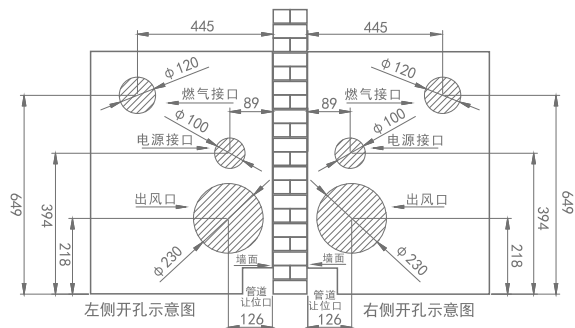
(图一 橱柜左右开孔图)
