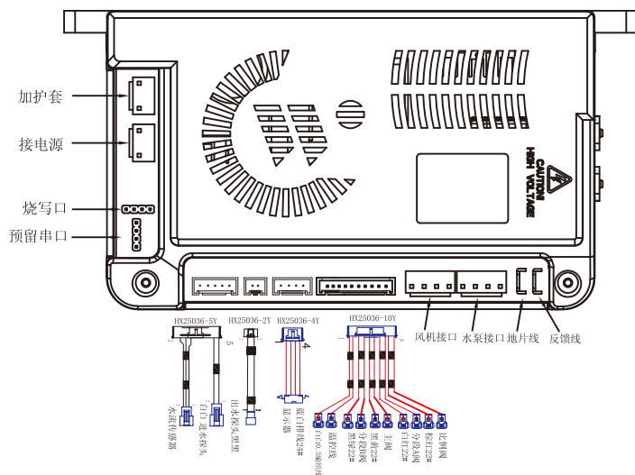
普恒温机控制器接线图
