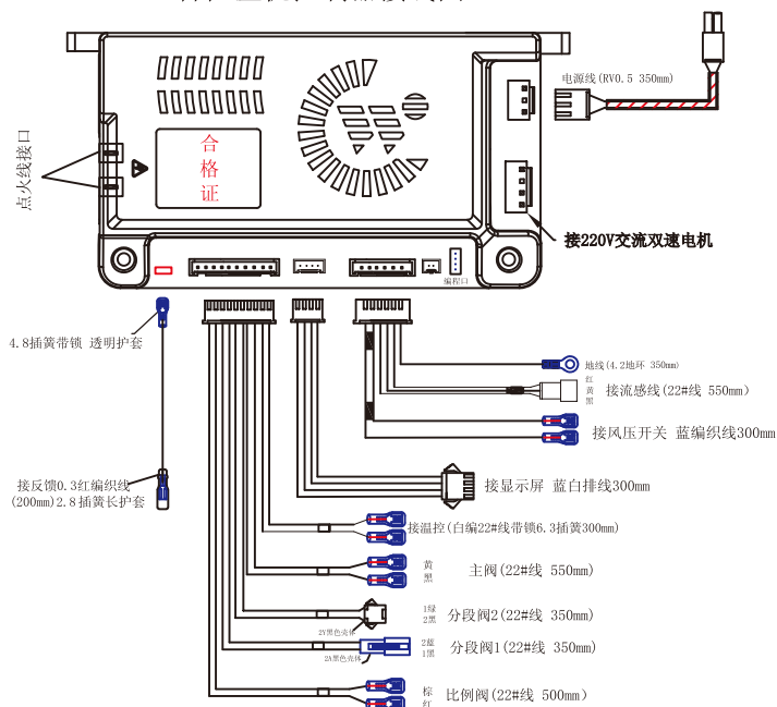
普恒温机控制器接线图
