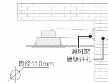
墙壁开孔形状及尺寸
