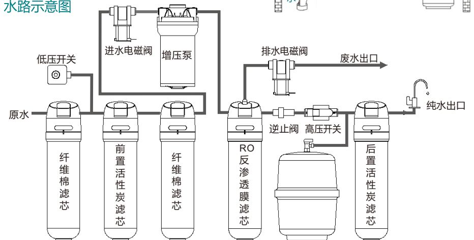
水路示意图
